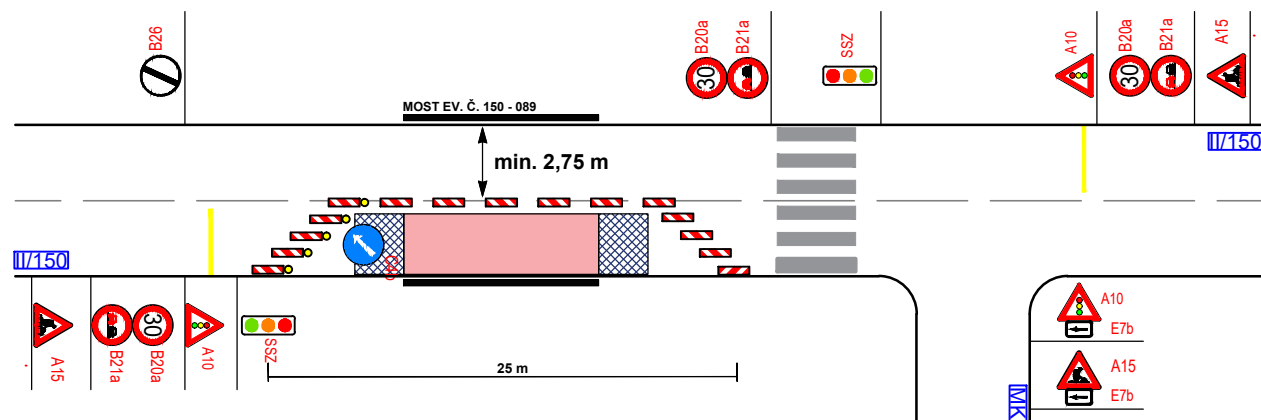
PRACOVNÍ MÍSTO - MOST EV. Č. 150 - 089 - ČÁSTEČNÁ UZAVÍRKA - ČÁSTEČNÁ UZAVÍRKA - SSZ - PRACOVNÍ MÍSTO V DĚLCE MAX. 25 m
