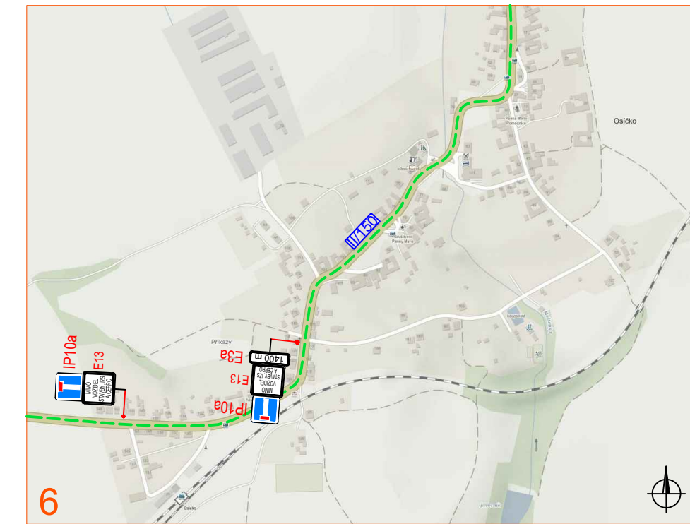
PRACOVNÍ MÍSTO - MOST EV. Č. 150 - 089 - ČÁSTEČNÁ UZAVÍRKA - ČÁSTEČNÁ UZAVÍRKA - SSZ - PRACOVNÍ MÍSTO V DĚLCE MAX. 25 m
